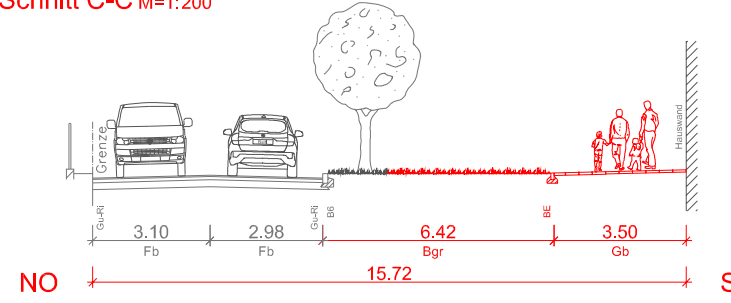
Schnitt C-C M=1:200
