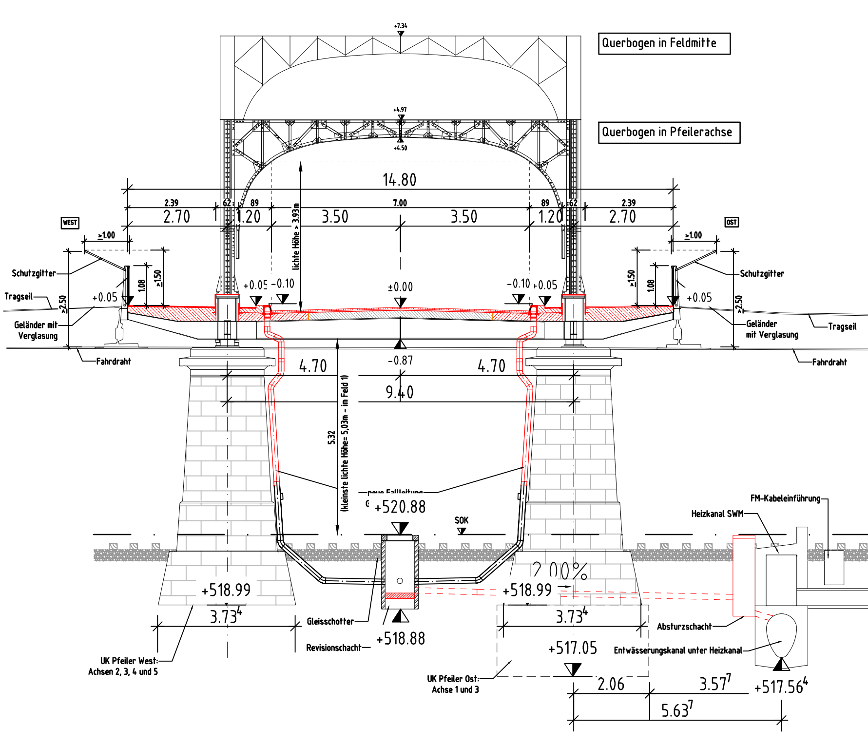
QUERSCHNITT AUFLAGERQUERTRÄGER IN PFEILERACHSE M 1:100 Entwässerung
