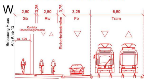
Abb. 2: Schematische Darstellung Querschnitt Am Knie mit Zweirichtungsradweg auf Höhe Hausnummer 11/13 (Quelle LHM)
